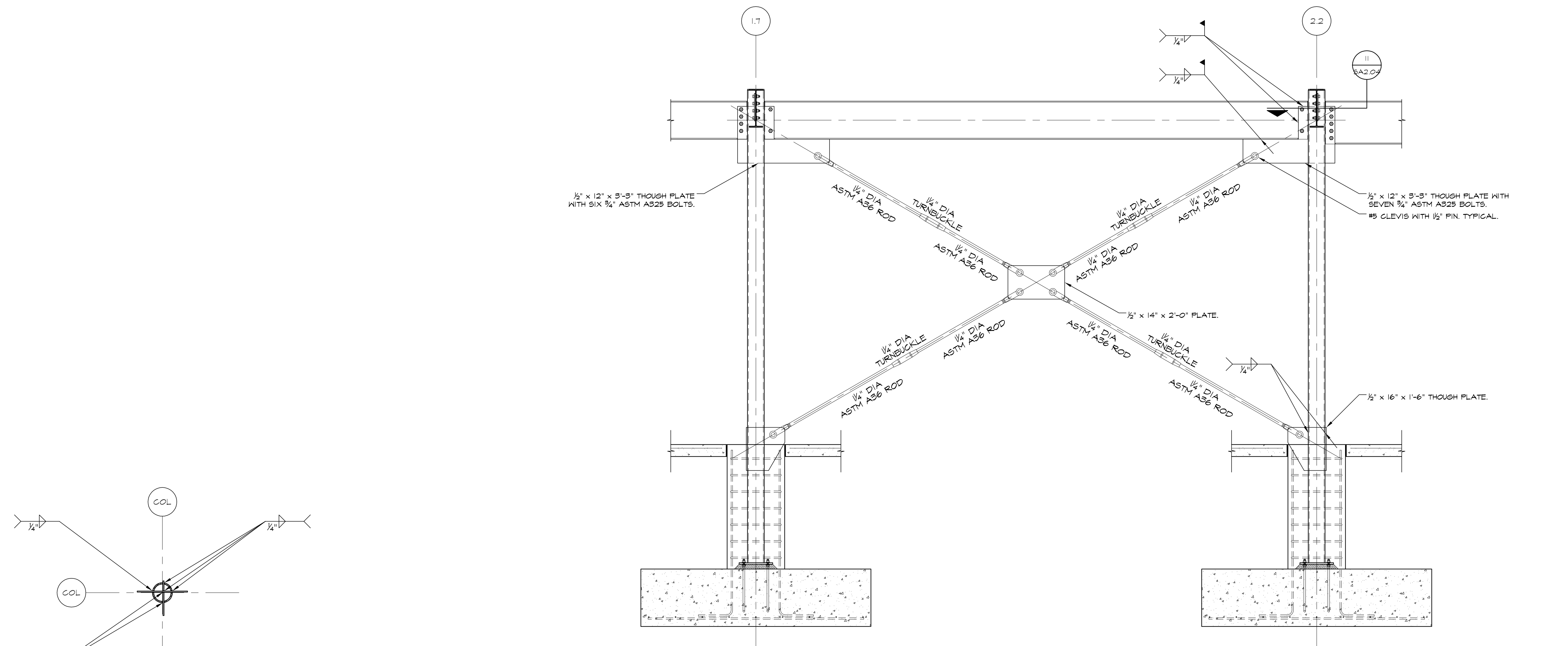
1 Section SCALE: 1/2" = 1'-0"
